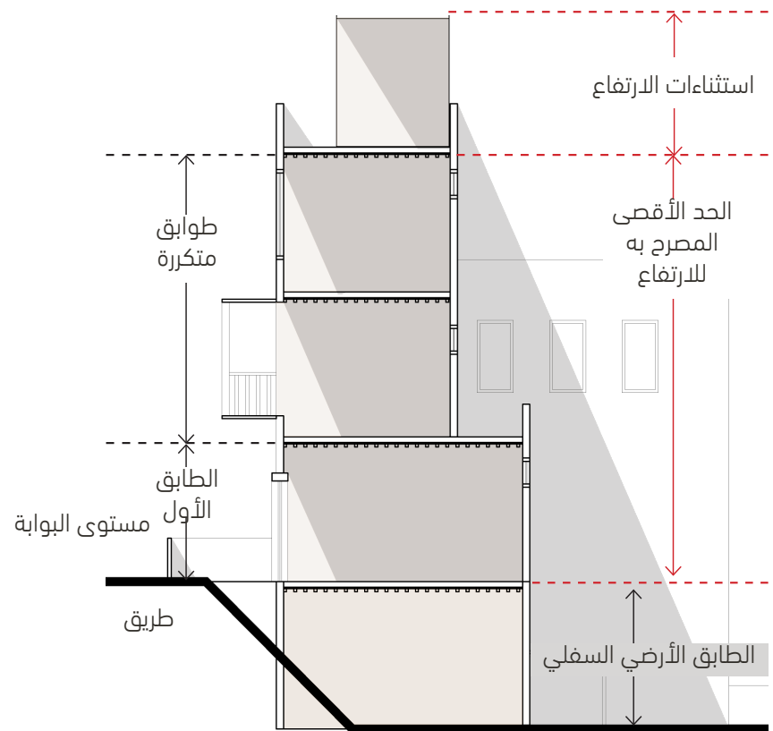
الشكل ١٢: حسابات ارتفاع المبنى
