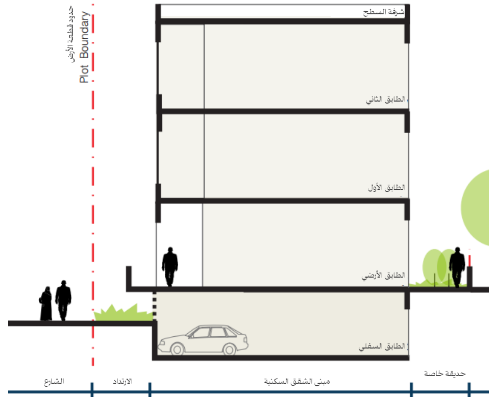
الشكل ٢١: مقطع عرضي يوضح نهج شبه الطابق السفلي
