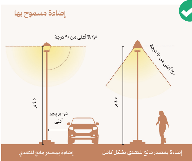
الشكل ٢: مثال على الإضاءة المانعة للتعدي والمانعة للتعدي بالكامل
