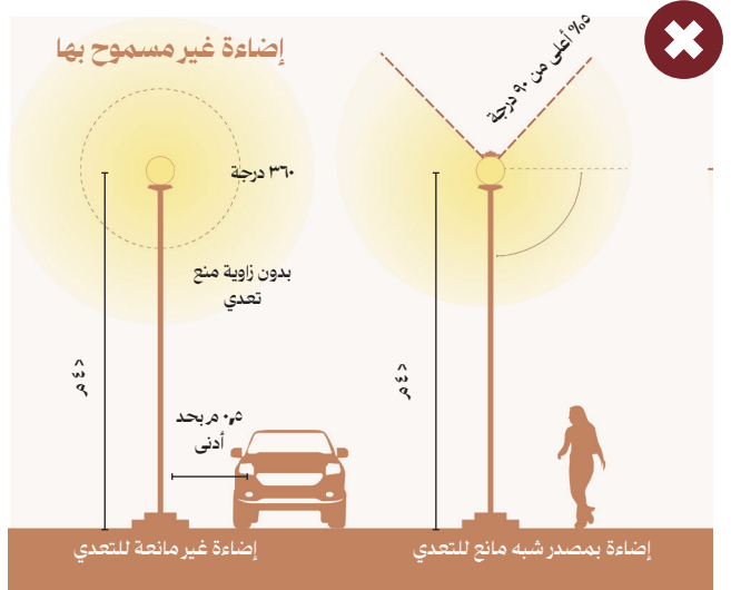
الشكل ١: مثال على تركيبات الإضاءة الغير مانعة للتعدي والإضاءة شبه مانعة للتعدي
